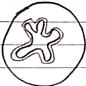
ATACTOSTELE
