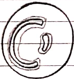
SIPHONOSTELE
